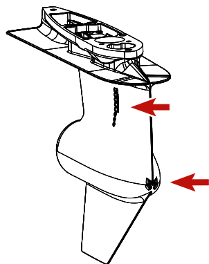
Doppelter Wassereinlass
